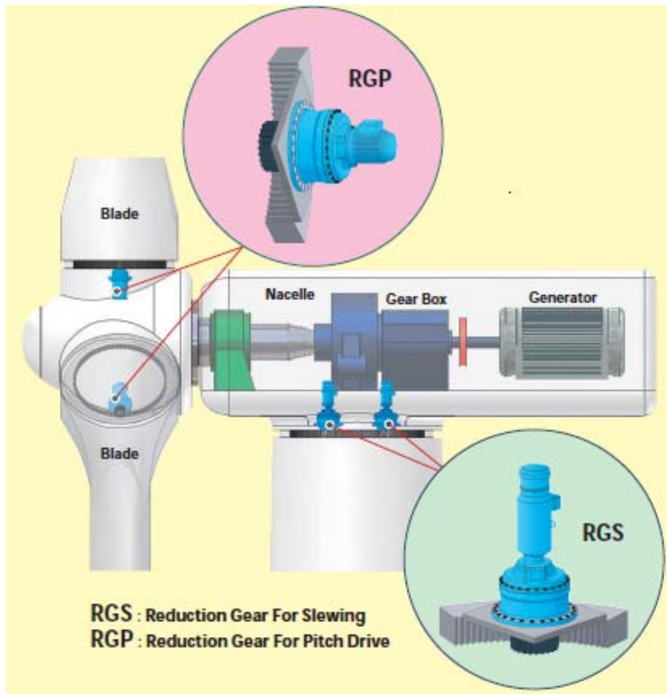
YAW 駆動装置(RGS シリーズ) PITCH 駆動装置(RGP シリーズ)
