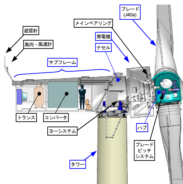
図1 J82の構成図
