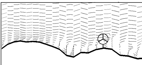
吹上・乱れ対策検討例（流れ解析）
